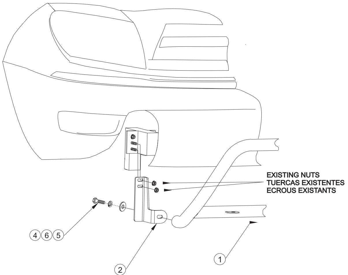
FIGURE 1 FIGURA 1 FIGURE 1 INSTALLATION VIEW OF PASSENGER SIDE, DRIVER SIDE OPPOSITE VISTA DE LA INSTALACIÓN DEL LADO DEL ACOMPAÑANTE OPUESTO AL LADO DEL CONDUCTOR VUE DU MONTAGE DU COTE PASSAGER, COTE CONDUCTEUR EN FACE
