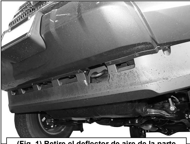
(Fig. 1) Retire el deflector de aire de la parte inferior del parachoques
