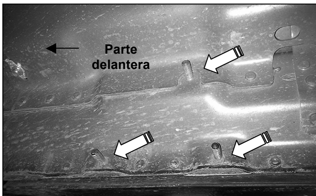
(Fig. 1) Ubicación del montaje delantero del lado del pasajero
