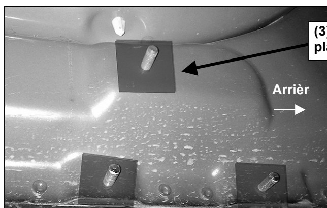
(Fig. 3) Enfiler des rondelles en plastique sur tous les goujons de montage. L'illustration montre l'emplacement de montage arrière côté passager
