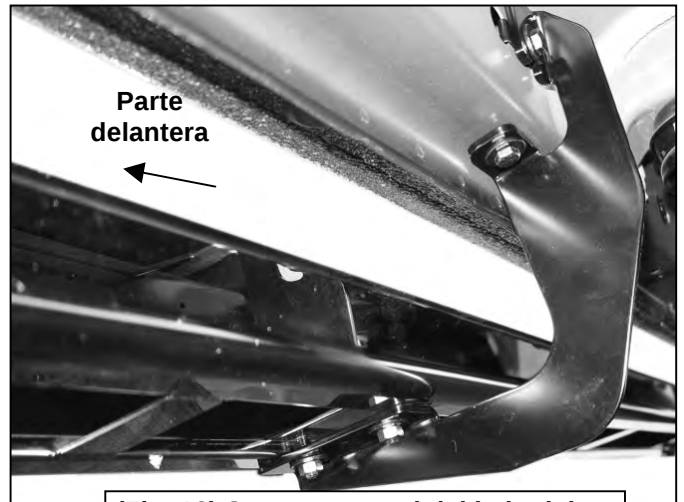
(Fig. 12) Soporte central del lado del pasajero sujetado al estribo lateral
