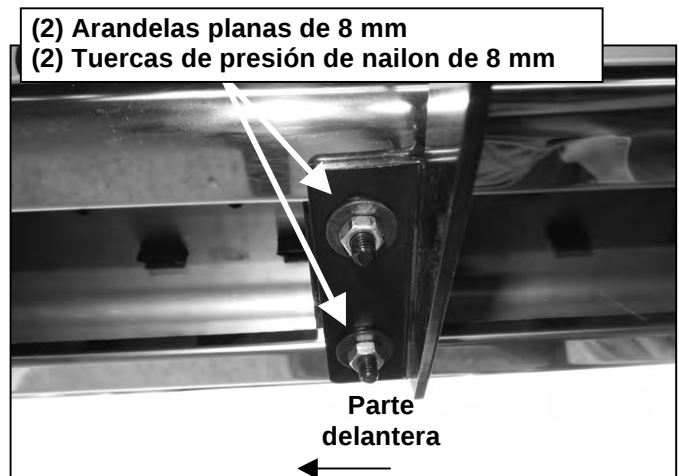
(Fig. 10) Conecte el estribo lateral al soporte
