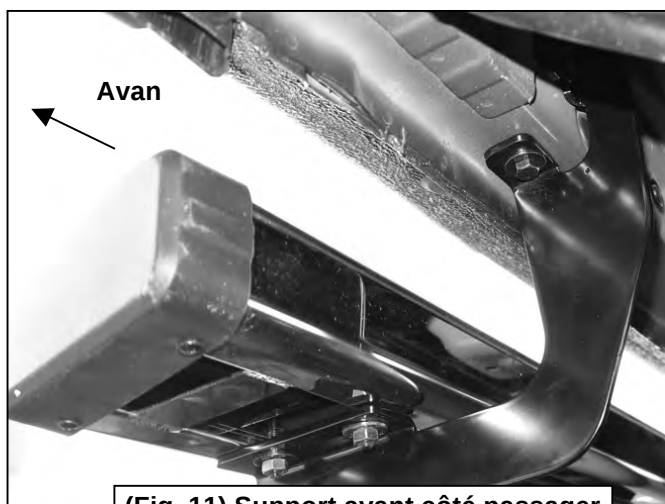
(Fig. 11) Support avant côté passager fixé au marchepied
