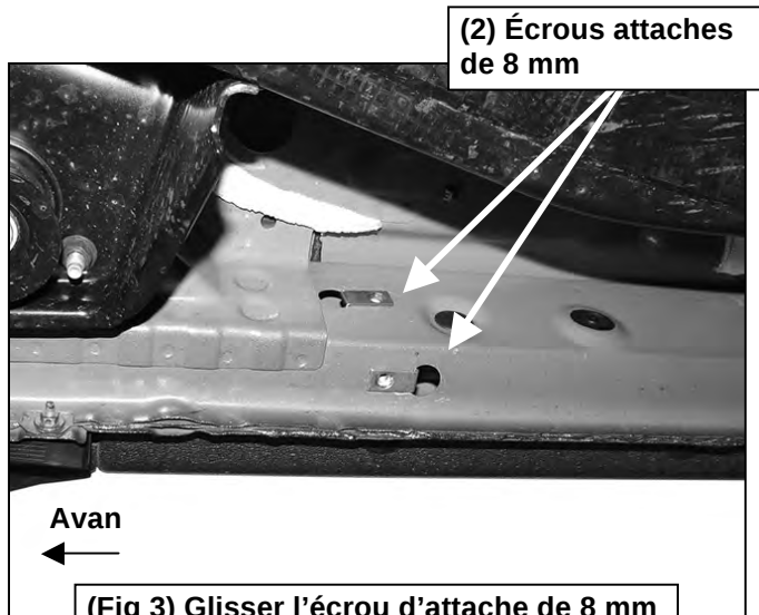
(Fig 3) Glisser l'écrou d'attache de 8 mm dans le grand trou et par-dessus le petit
