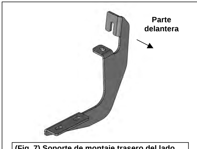
(Fig. 7) Soporte de montaje trasero del lado del pasajero
