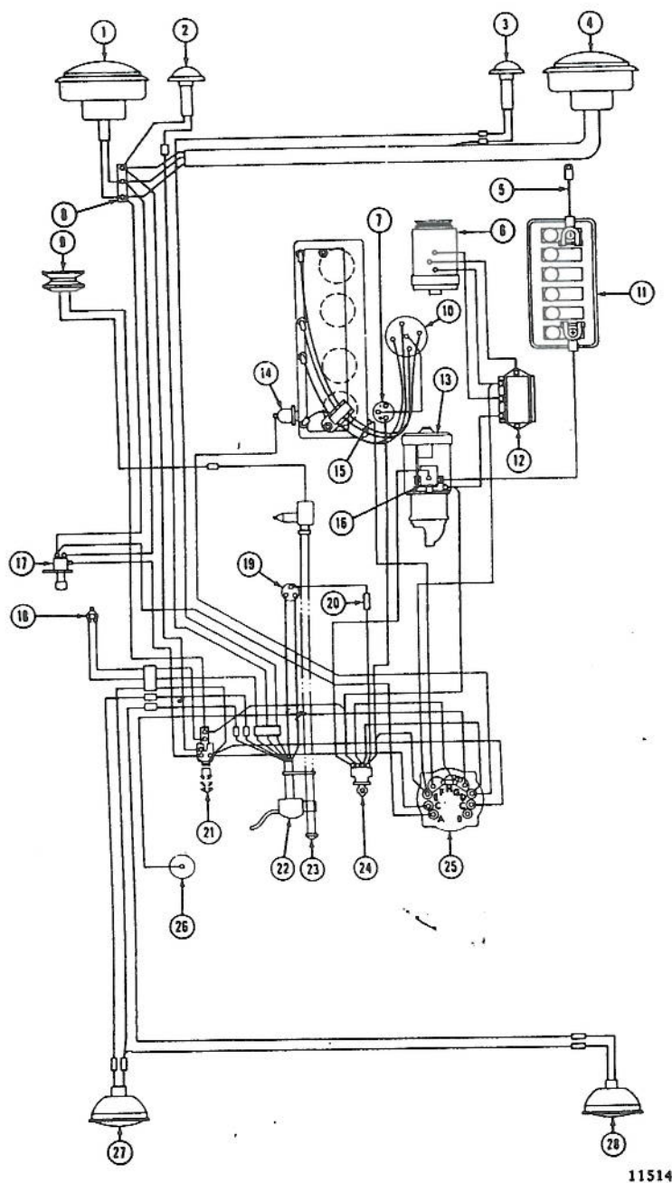
FIG. 144—WIRING DIAGRAM—MODEL CJ-3B
